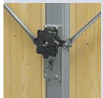
Innengriff, Profilzylinder-Schloss, Verriegelungsstangen, im Geräteraum
